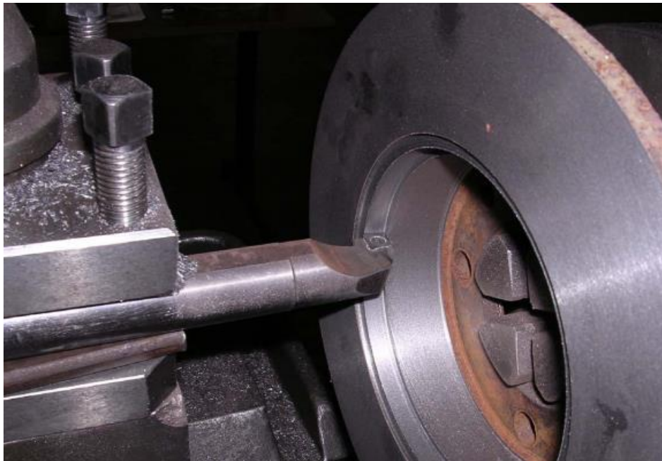
Slika 3.3. Uzdužno unutarne tokarenje [8]
