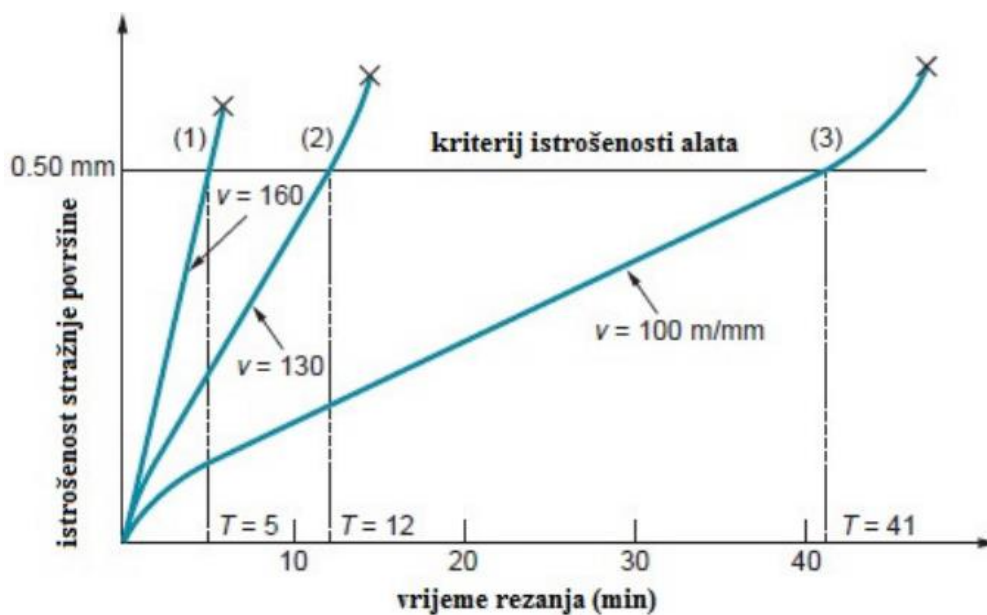
Slika 4.5. Utjecaj tri različite brzine rezanja na trošenje stražnje površine [13]
