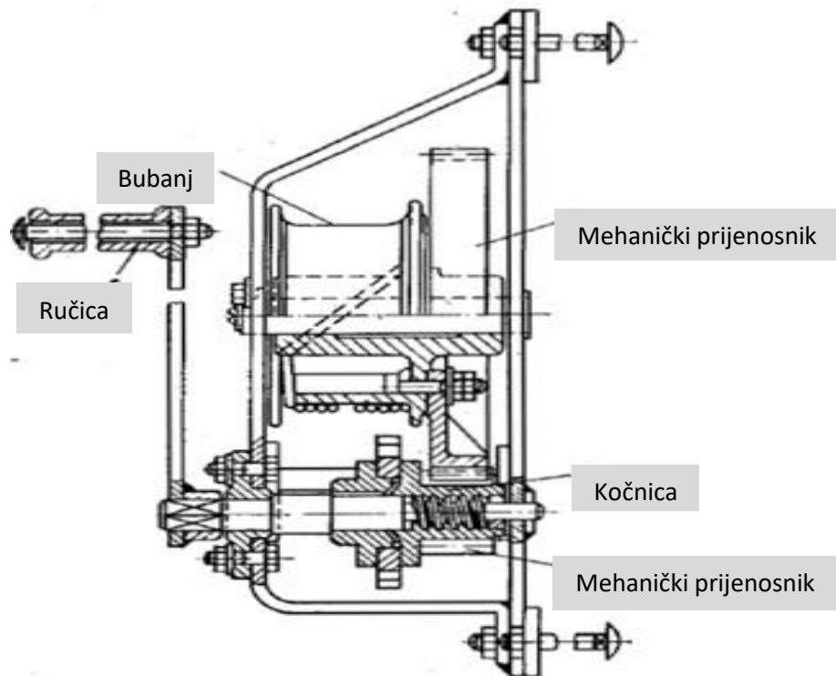
Slika 2.16 Zidno vitlo
