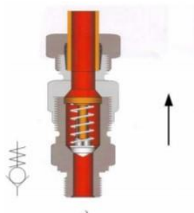
Slika 8.10 Presjek nepovratnog ventila s oprugom
