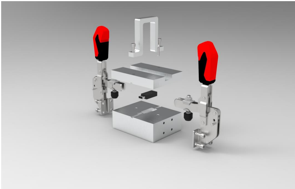
Slika 23. Render kalupa
