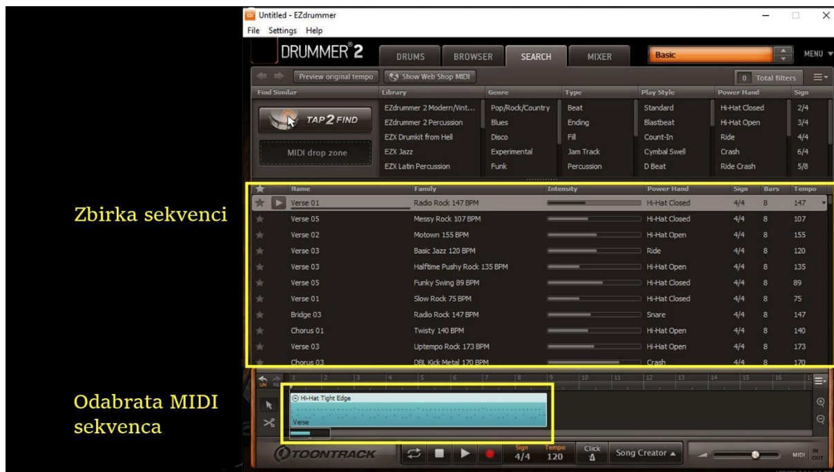
Slika 3.1.2. EZdrummer software
