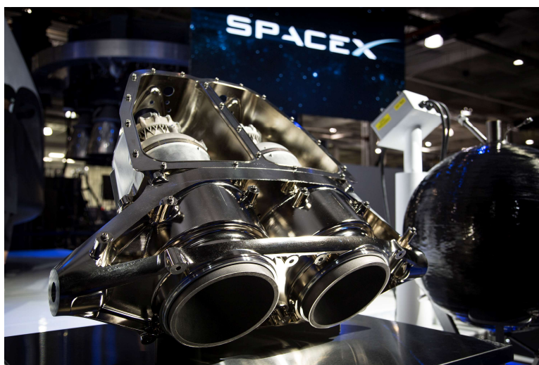
Slika 4.3 Raketni motor tvrtke SpaceX proizveden 3D ispisom [26]
