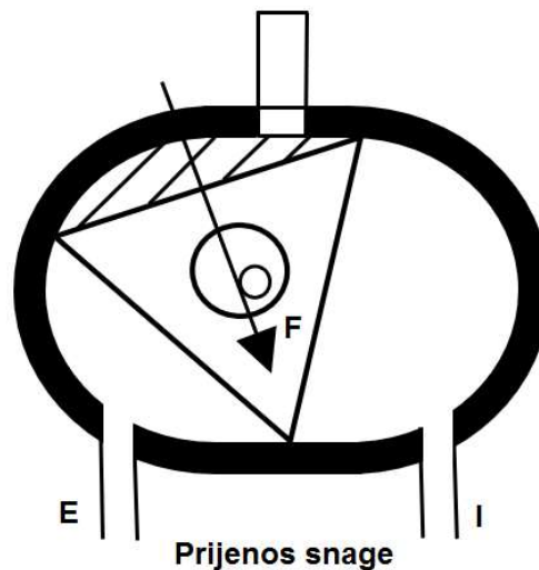
Slika 3.7 Shematski prikaz prijenosa snage [11]
