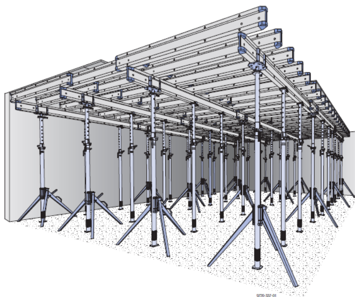
Slika 4.13. Slika 4.13. Oplati sustav Dekaflex [6]
