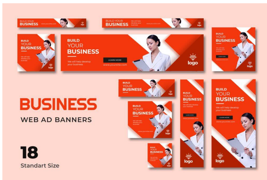
Slika 8. Primjeri bannera
