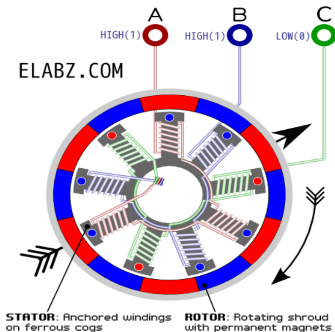
Slika 2.6- konstrukcija trofaznog BLDC motora[14]
