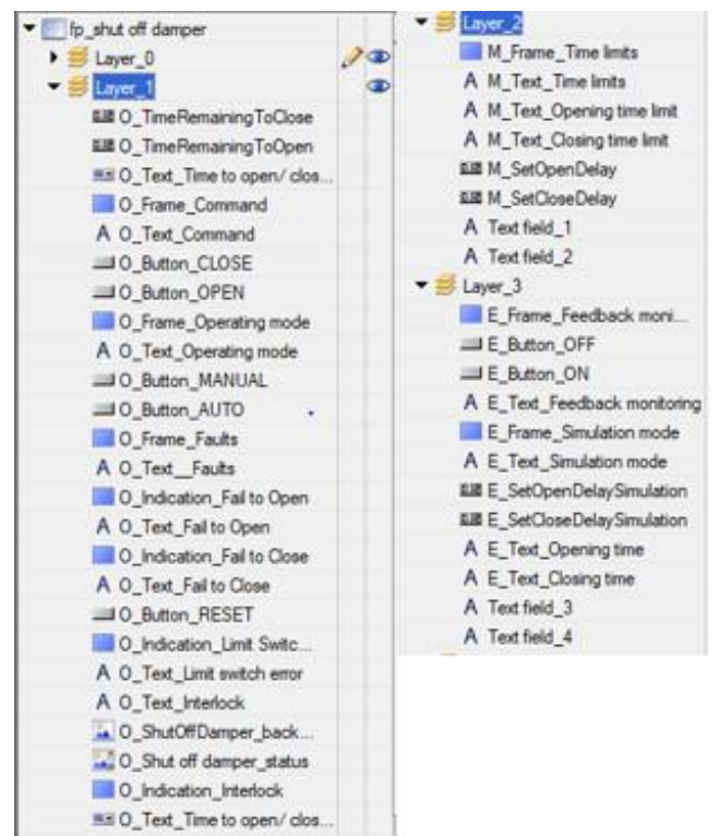
Slika 23 Slojevi faceplatea
