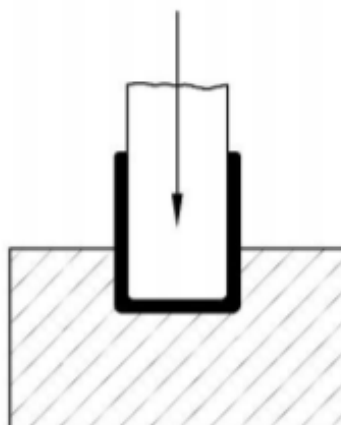
Slika 9. Savijanje lima u U profil [15]
