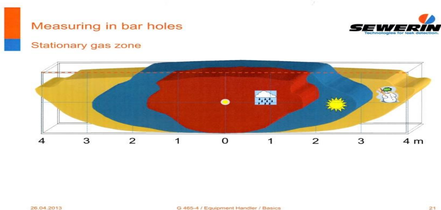
Slika 4.7 Stacionarna zona plina pod različitim vremenskim uvjetima [8]
