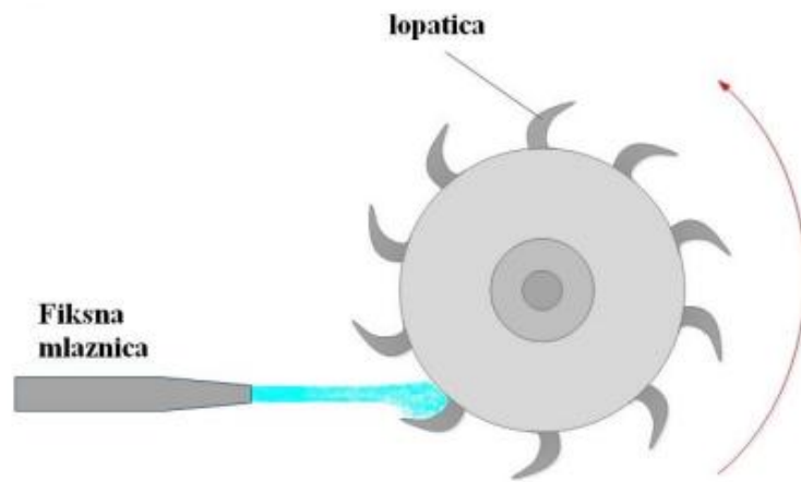
Reakcijska turbina
