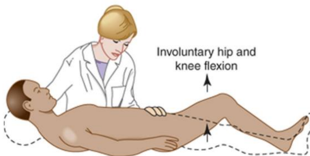
Slika 3.3.2. Brudzinskijev znak
