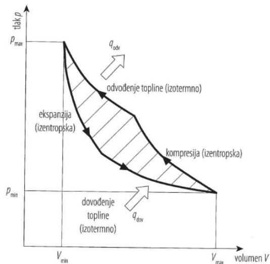
Slika 2.1 p-V dijagram idealnog lijevokretnog Carnotovog procesa [1]
