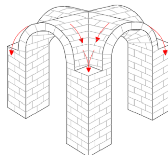
križni svod
