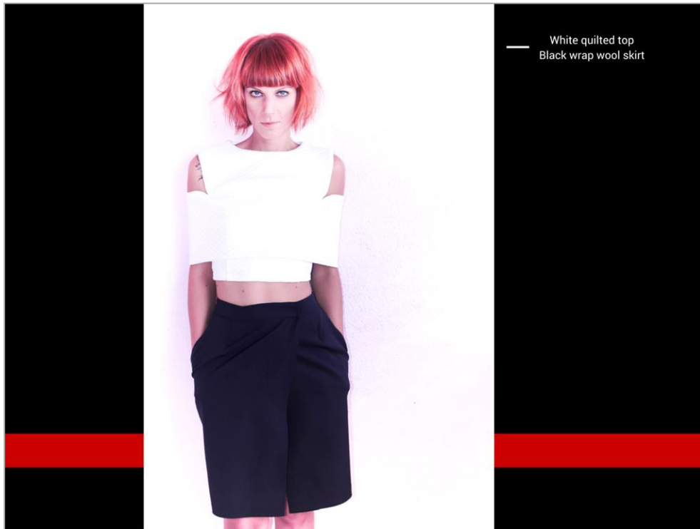
Slika 8.4. Katalog
