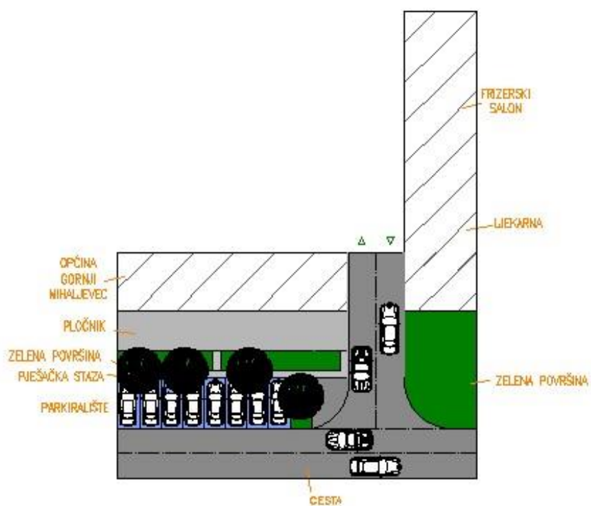
Slika 19. Prijedlog sanacije [18]
