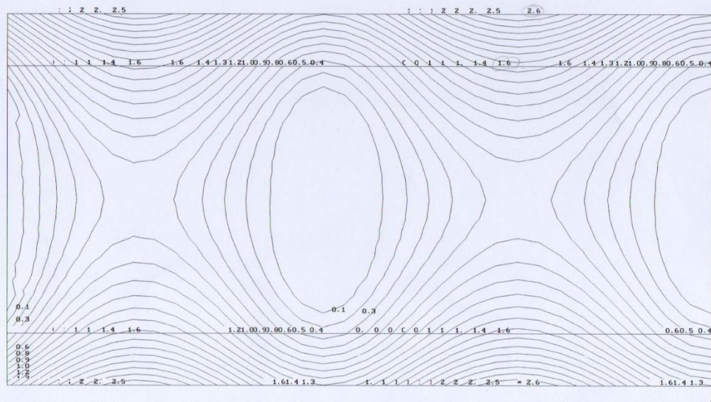
Slika 15. Numerički model: pomaci rasponskog sklopa uslijed djelovanja dodatnog stalnog opterećenja
