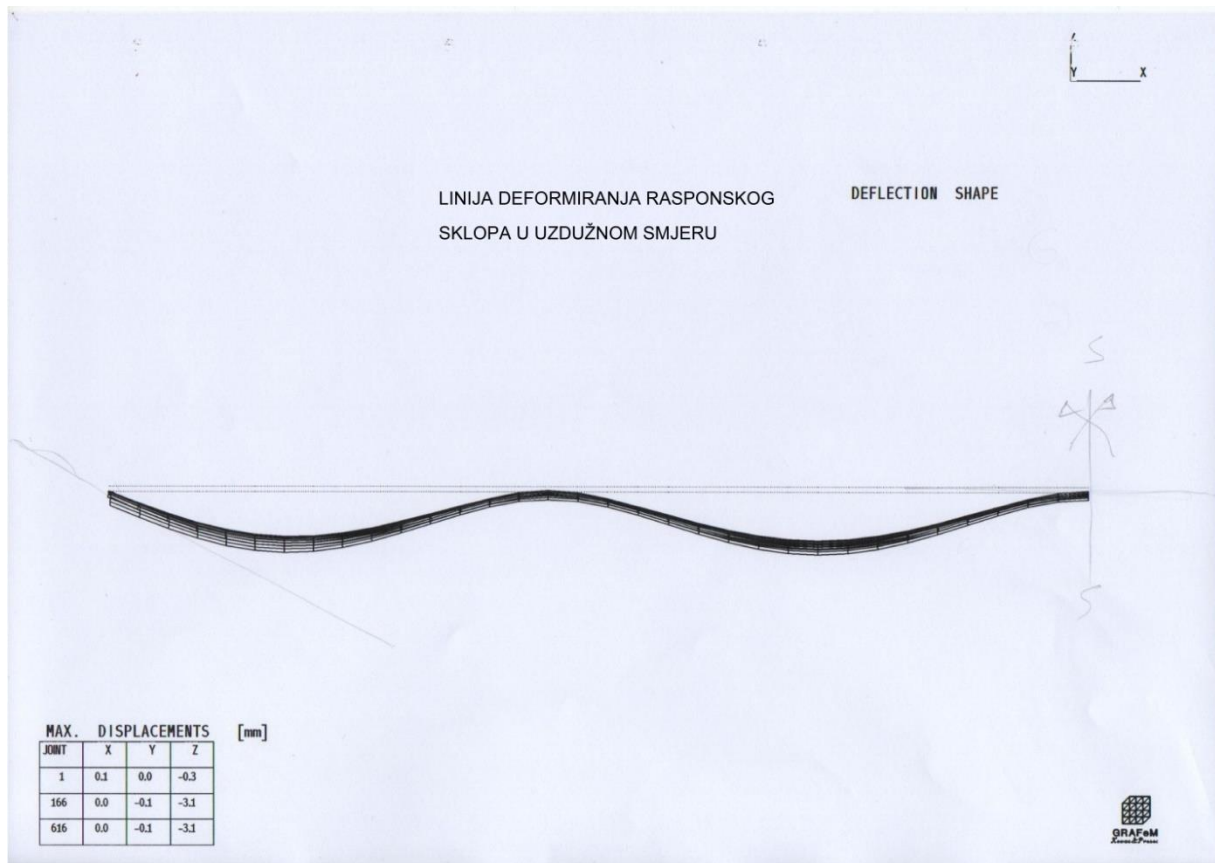
Slika 11. Numerički model: linija deformiranja rasponskog sklopa uslijed djelovanja vlastite težine
