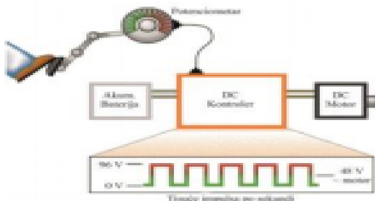
Slika 3.5. Prikaz načina rada kontrolera u elek.automobilu
