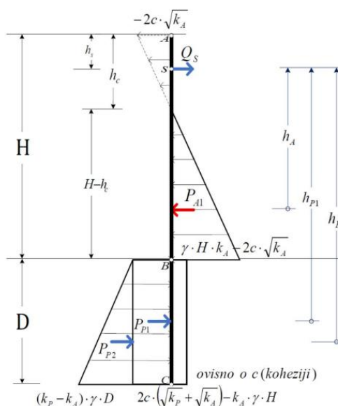
Slika 4.4. Sile usidrene zagatne stijene.
