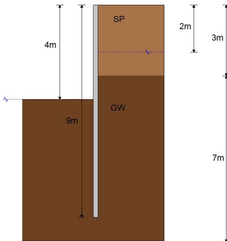
Slika 5.15. Poprečni presjek idejnog rješenja.
