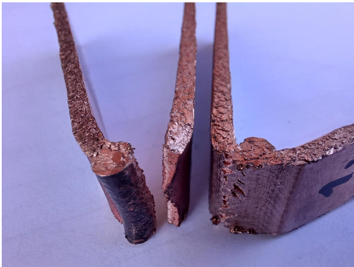
Slika 52. Epruvete prvog uzorka
