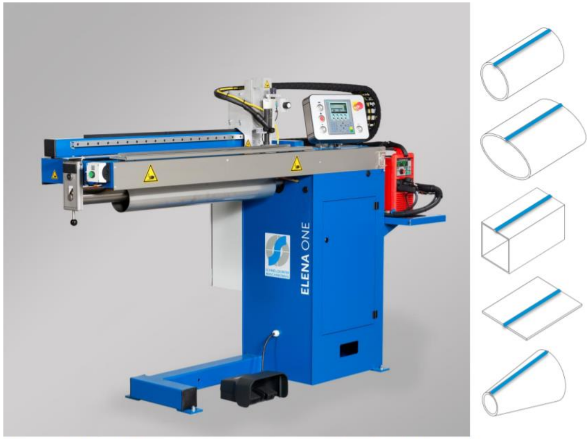
Slika 25. Prikaz Semac Elena One automata i primjera mogućih zavarivanja cijevi
