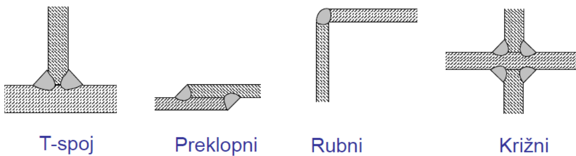
Slika 17. Primjeri kutnih spojeva [37]
