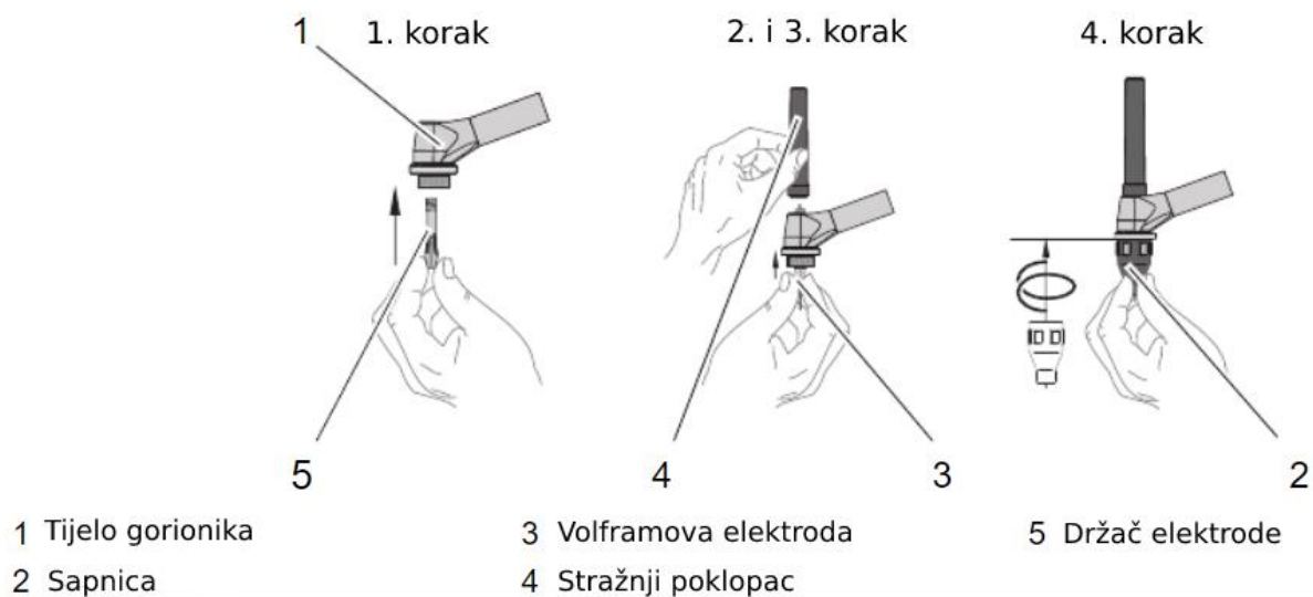
Slika 38. Prikaz postavljanja elektrode u gorionik [31]
