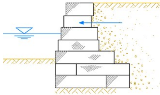
Slika 3.14 Gabionski madraci i košare - elementi vertikalne gravitacijske konstrukcije obaloutvrde [7]
