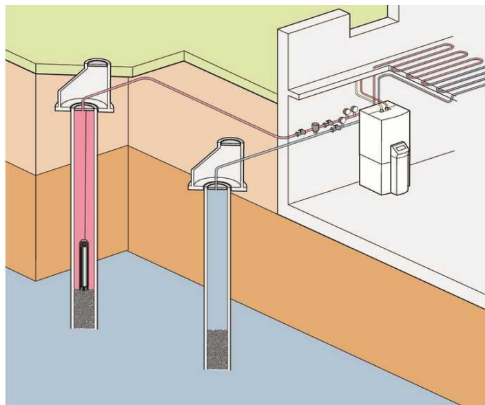
Slika 7.2.3 Dizalica topline podzemnih voda [39]
