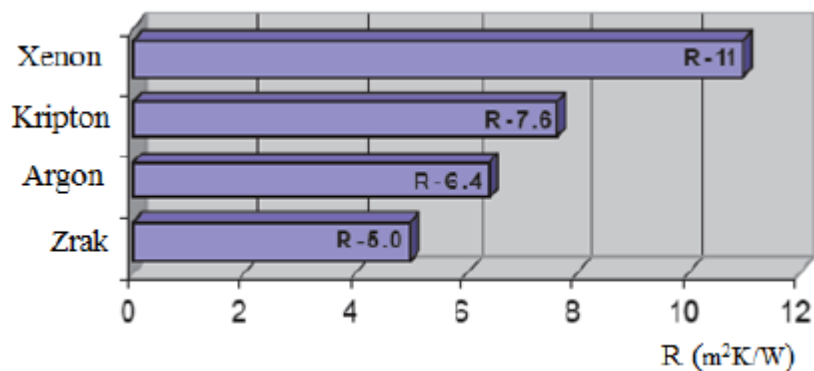
Slika 4.5.2.1 Toplinski otpor GFP-a s različitim plinovima [25]
