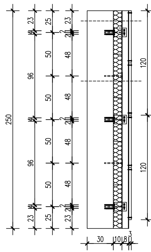
PRESJEK
