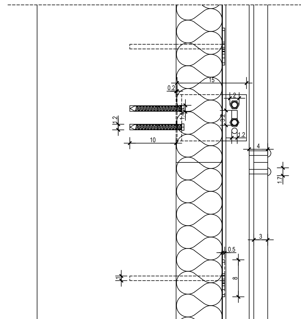
PRESJEK DETALJ 1:5
