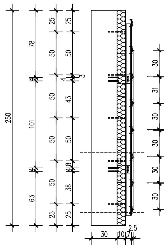
PRESJEK
