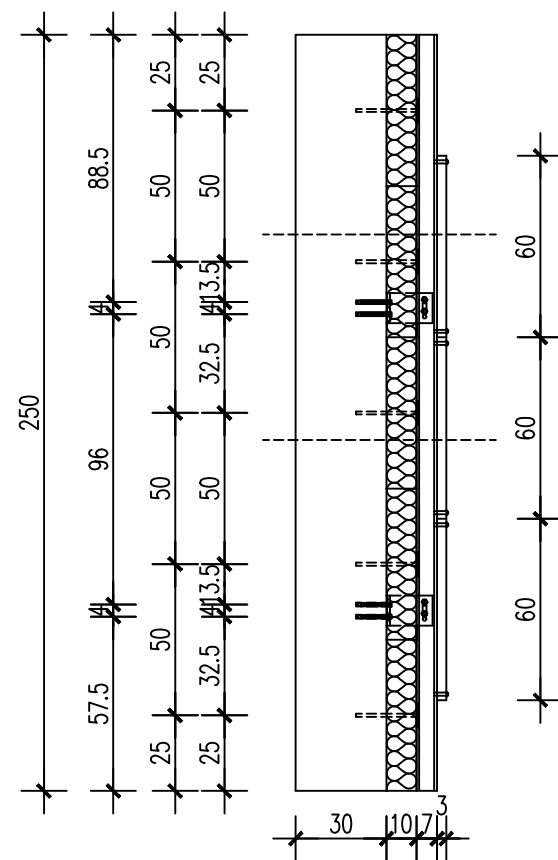
PRESJEK
