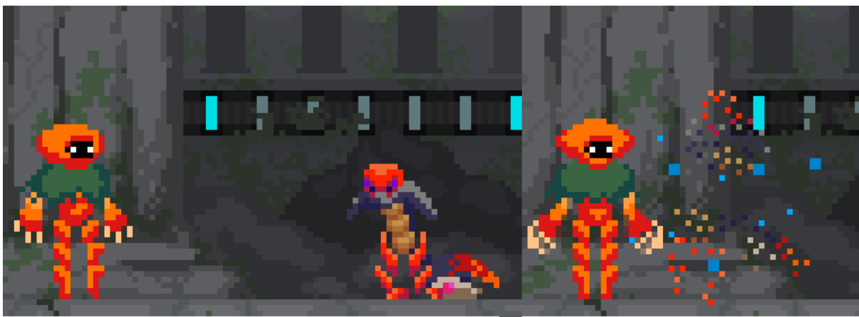
Slika 4.3.15. Nestajanje neprijatelja
