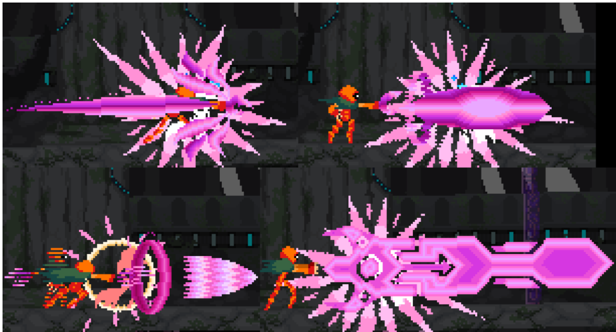
Slika 4.2.16. Finisher napadi
