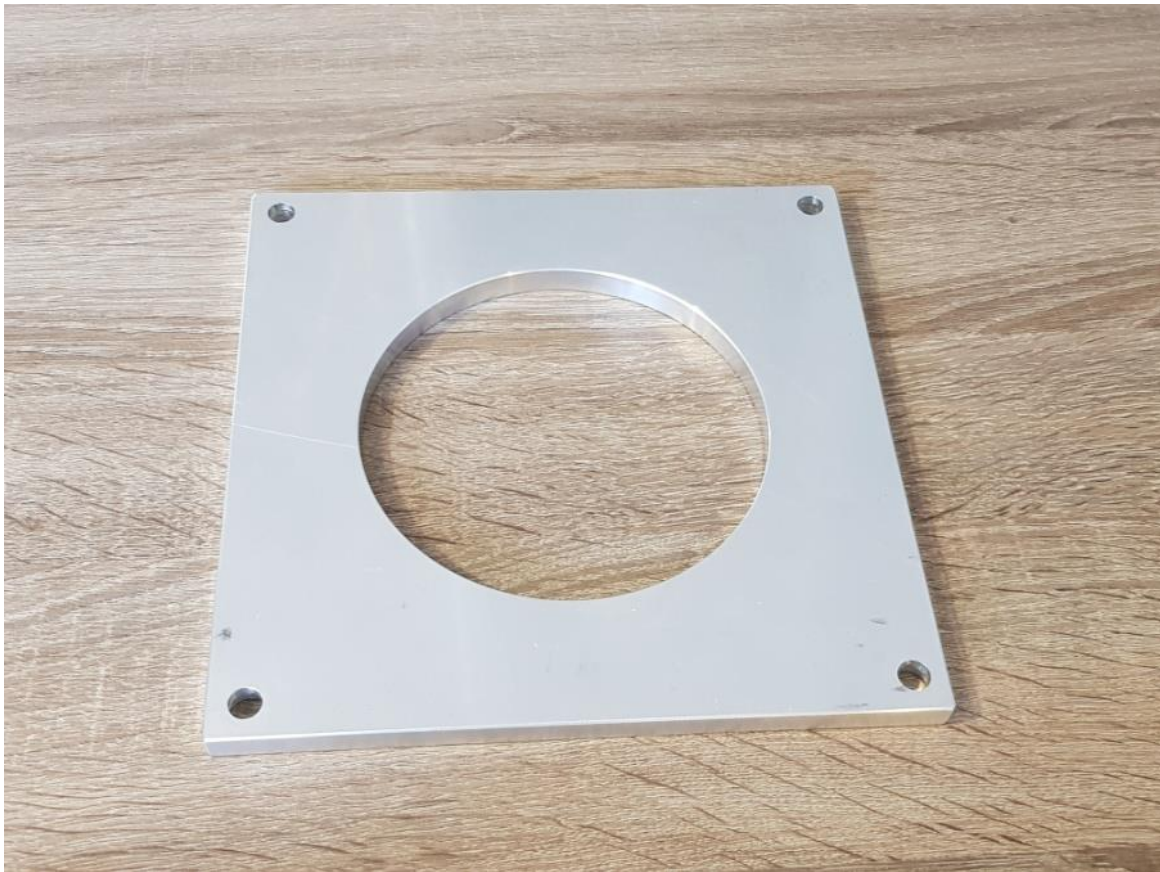
Slika 20. Stezna ploča
