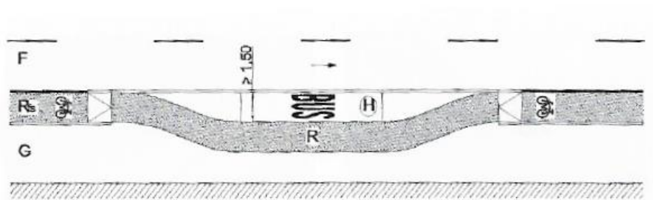
b) prijelaz biciklističkog traka u biciklističku stazu pokraj stajališta
