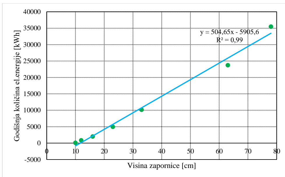
Slika 57. Grafički prikaz ovisnosti količine proizvedene el. energije o visini zapornice
