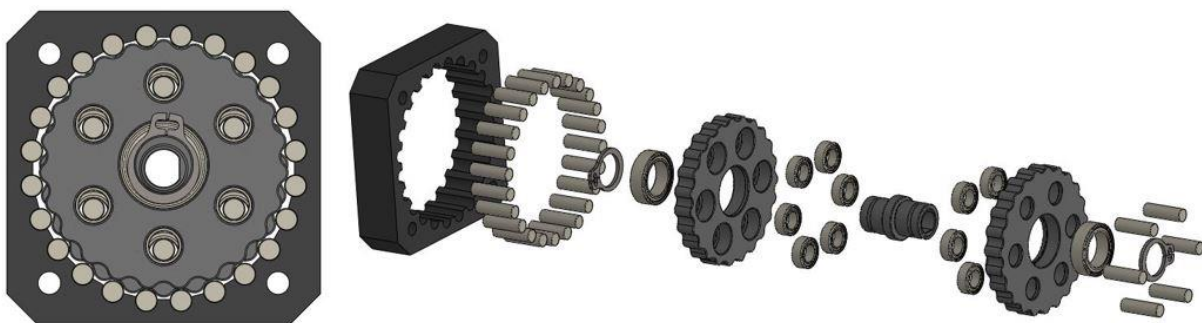
Slika 21. Model cikloidnog reduktora šestog zgloba robotske ruke
