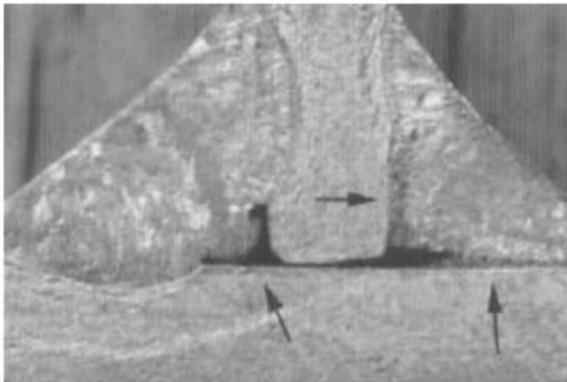
Slika 3.10. Naljepljivanje u kutnom spoju [29]
