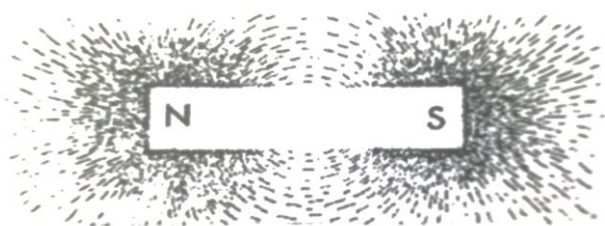
Slika 2.7. Magnetsko polje [17]
