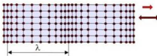
Slika 2.21. Širenje longitudinalnog vala [21]
