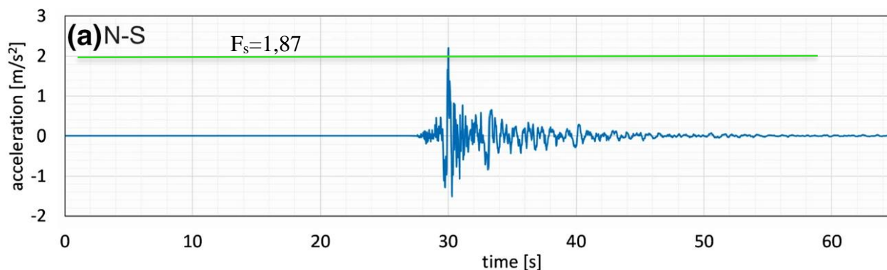
Slika 7.4.: Akcelorogram zagrebačkog potresa 22.03.2020. sa horizontalnim koeficijentom ubrzanja 0,23
