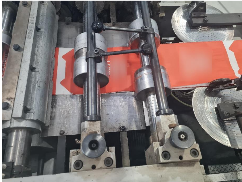
Slika 9.8. Sljepljivanje gornjeg dijela vrećice sa donjim pomoću longitudinalnog ljepliva na vučnim valjcima prije rezanja tijela
