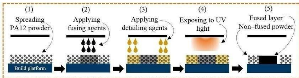
Slika 4.2.8 MJF tehnologija 3D tiska
