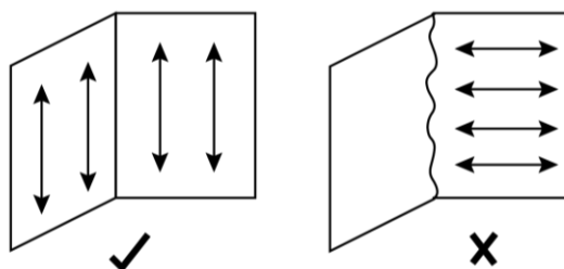
Slika 3.4 Prikaz pravilnog i nepravilnog toka vlakancu prilikom izrade projekta
