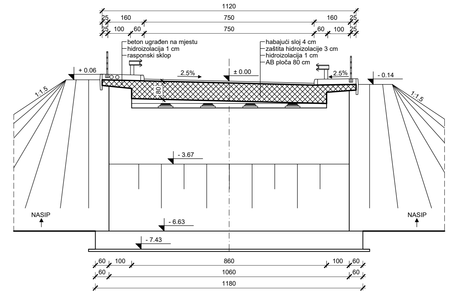
Poprečni presjek MJ 1:100
