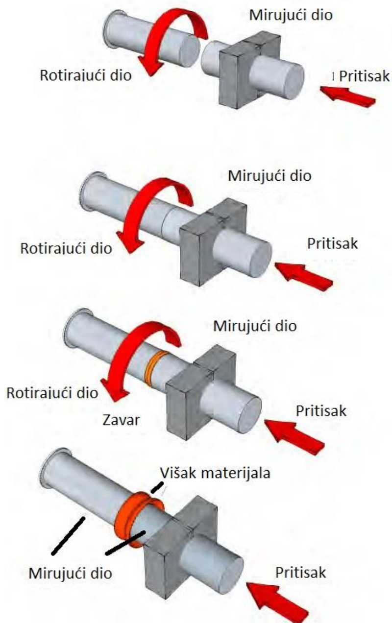
Slika 4.2 Shematski prikaz rotacijskog zavarivanja trenjem [10]
