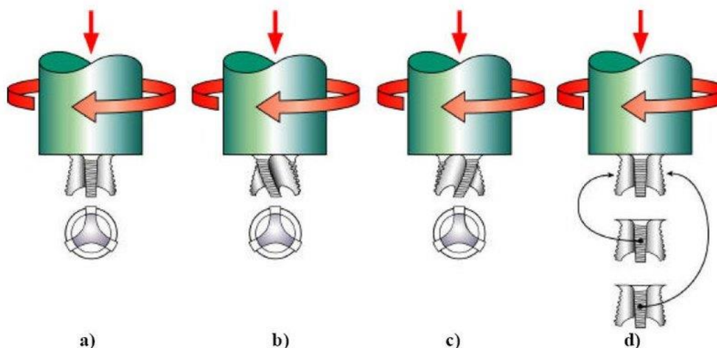
Slika 4.22 Flared-Triflute™, Prikaz različitih izvedbi navoja na trnu alata:
