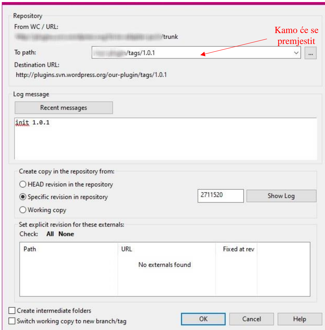
Slika 6.37 - Ažuriranje dodatka
