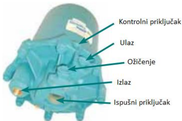
Slika 15. Sušilo zraka [1]
