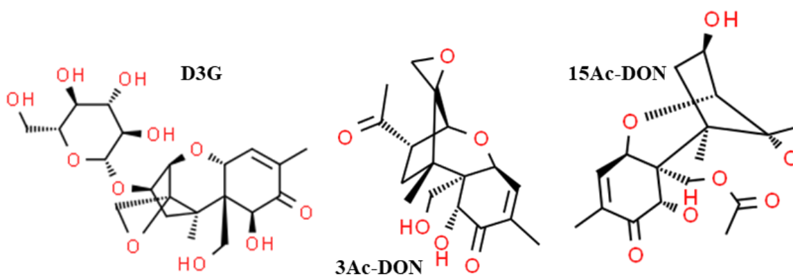
Slika 7. Strukturne formule modificiranih oblika DON-a.
