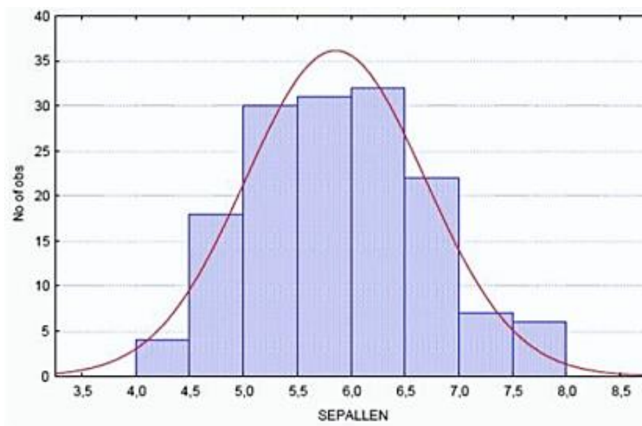
Slika 4 Primjer Histograma
