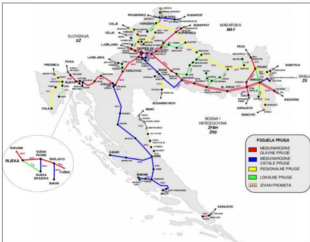
Slika 2. Željezničke pruge u Republici Hrvatskoj razvrstane prema gospodarskom značaju
