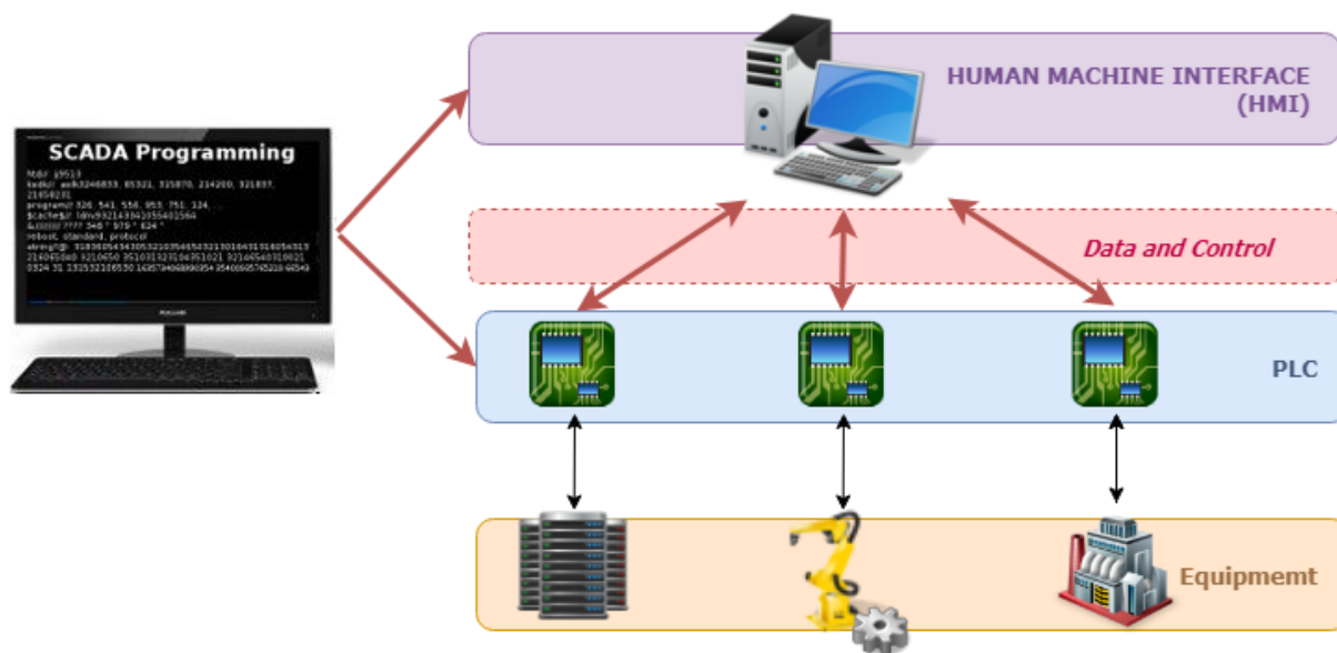
Slika 2. SCADA system
