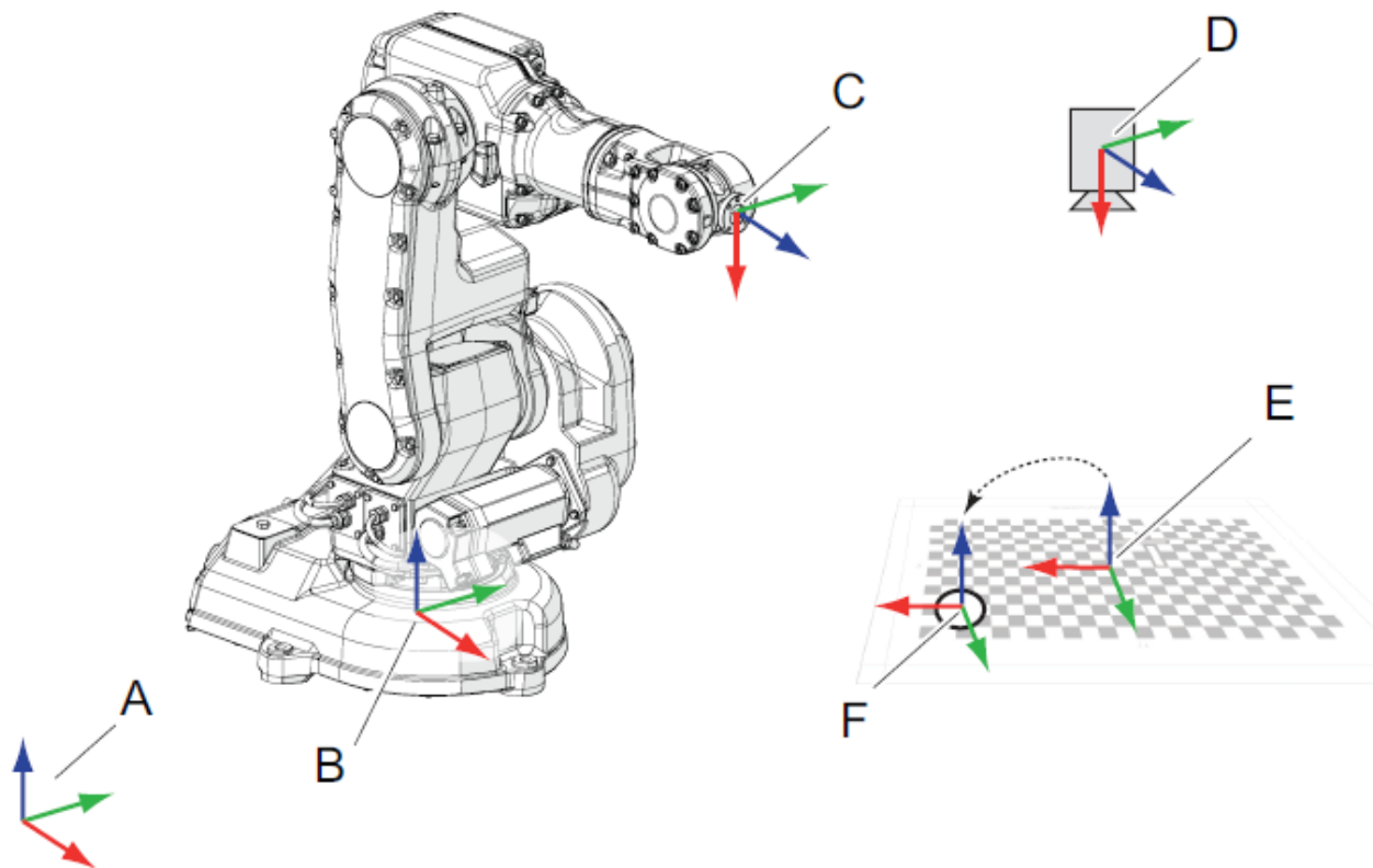
Slika 45 – Koordinatni sustavi robota[5]
