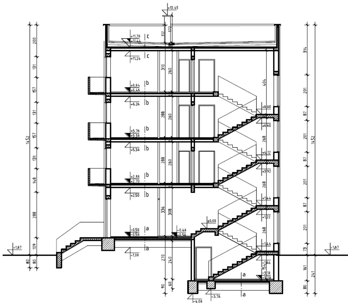
Slika 11 – Presjek MJ 1:100
