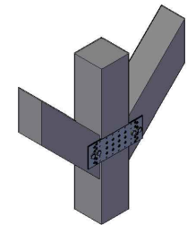
IZOMETRIJA 1:25
