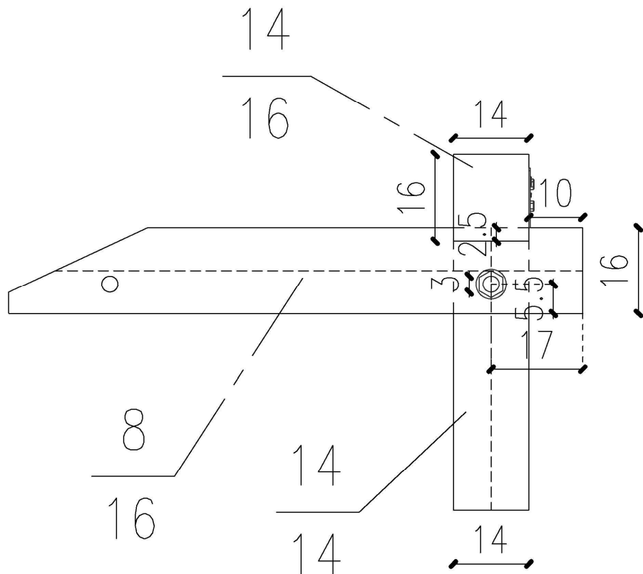
POPREČNI PRESJEK
