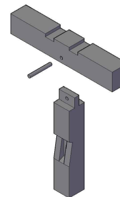
IZOMETRIJA 1:25
