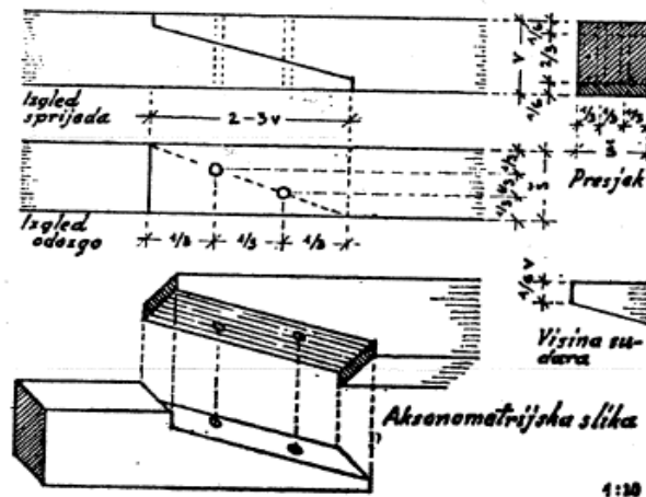
Slika 11. Kosi prijeklop s ravnim sudarima [1]
