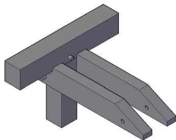
IZOMETRIJA 1:25
