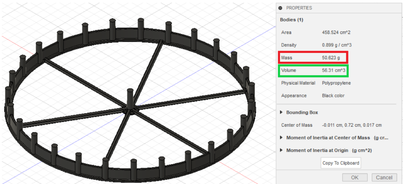
Slika 4.4.3. masa izrađenog 3D modela proizvoda [8]
